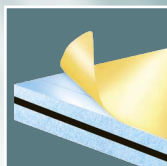
XPS-Innenkern (mit schalldämmender Schwerfolie)
