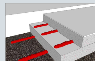
5 COSMO® PU-160.110 Adhesivo aislante
